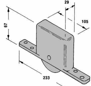
72-402 BOTTOM ROLLER
